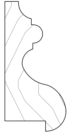
GCM14 1/8 x 2 3 / 8
