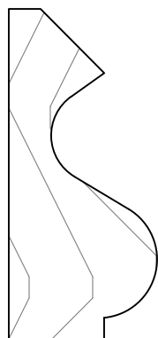
GCM2004 \frac{7}{8} X 1 \frac{15}{16}
