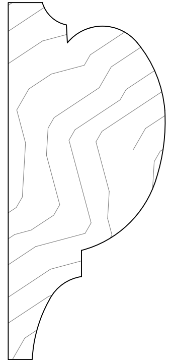
GCM6014 1 5/8 x 3 1/16
